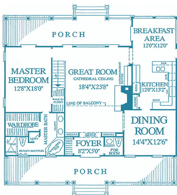
Größeres Country Cape Cod Cottage für die 2-Kind-Familie
